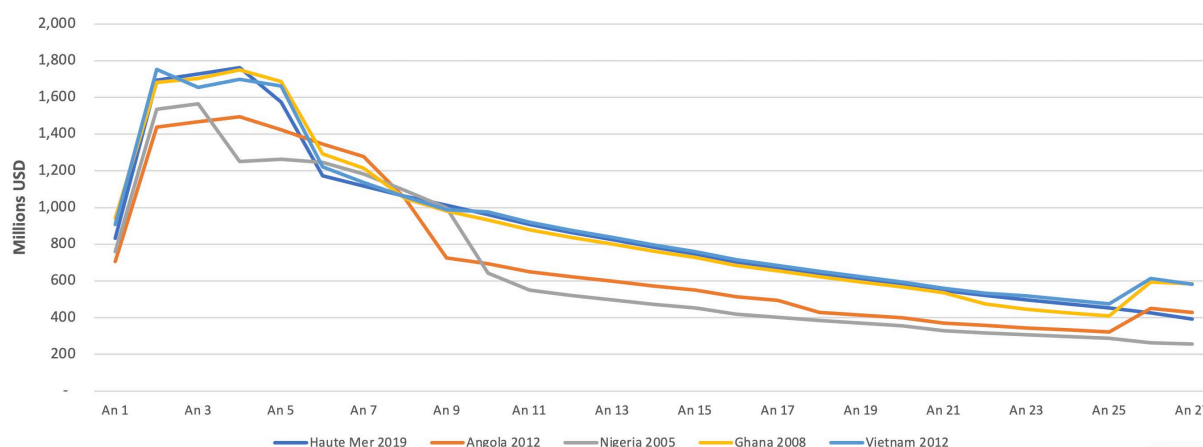
Figure 14: Revenus du droit du Contracteur après impôts (base de référence : 70 $/bbl)
