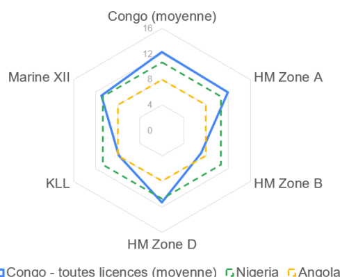
Figure 36 : Opex moyens 2016-2018 ($/boe)
