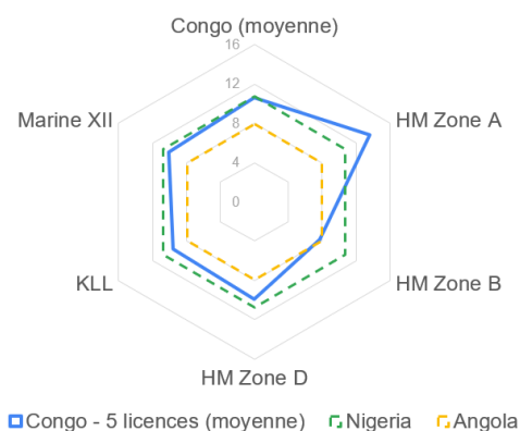
Figure 35 : Opex moyens 2013-18 ($/boe)
